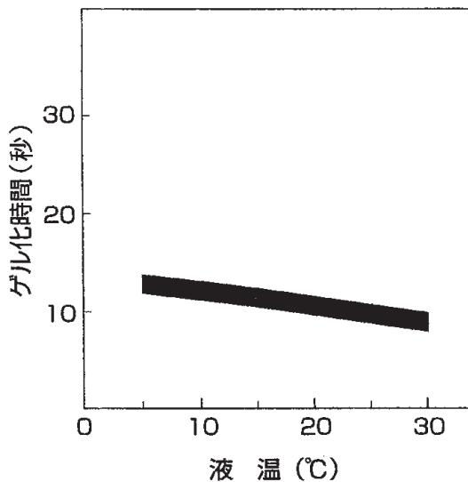
図-1 液温によるゲル化時間の変化
