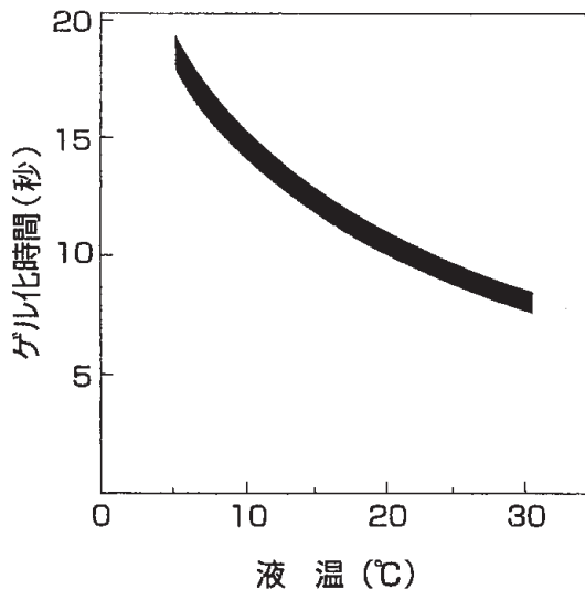
図-1 液温によるゲル化時間の変化
