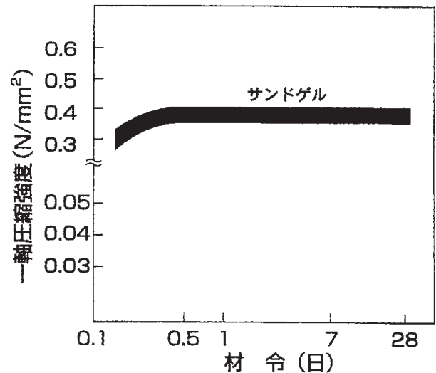
図-2 材令によるゲル強度の変化
