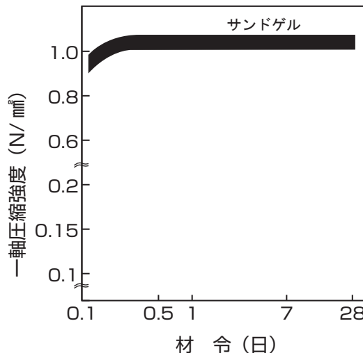
図-2 材令によるゲル強度の変化
