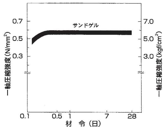
図-2 材令によるゲル強度の変化
